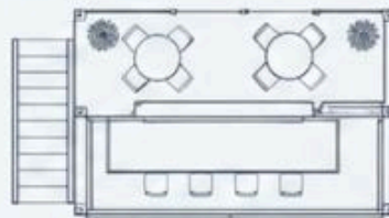
PLANTA / USO
